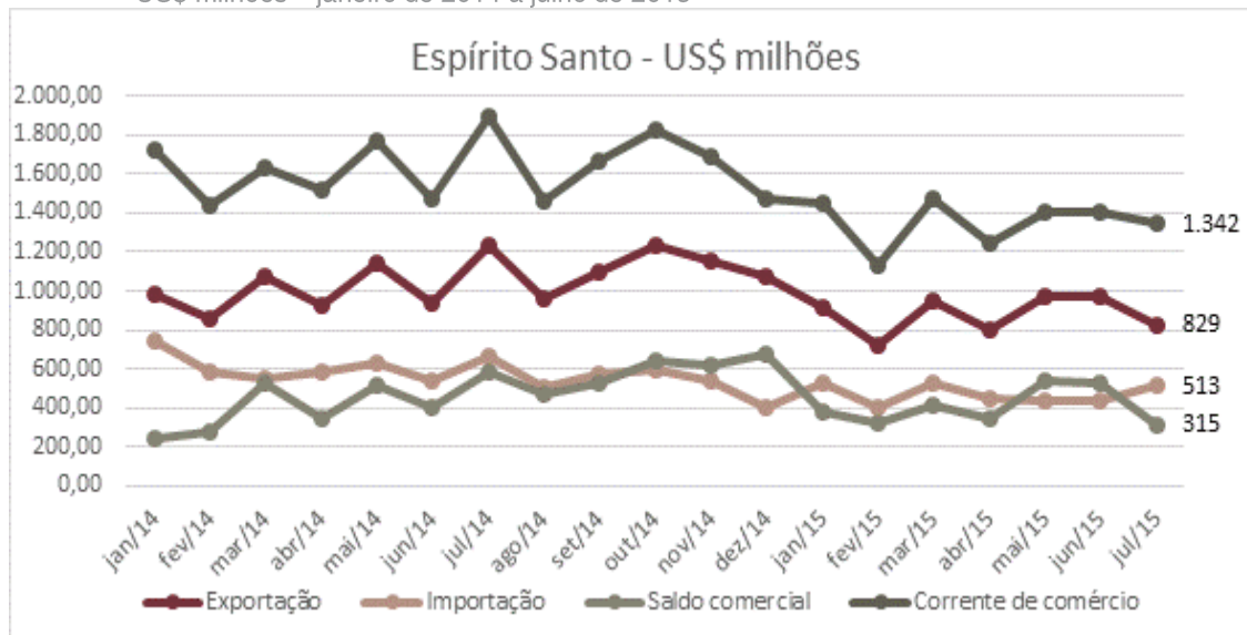
Gráfico 1 - Exportações, Importações, Saldo Comercial e Corrente de Comércio do Espírito Santo US$ milhões – janeiro de 2014 a julho de 2015
