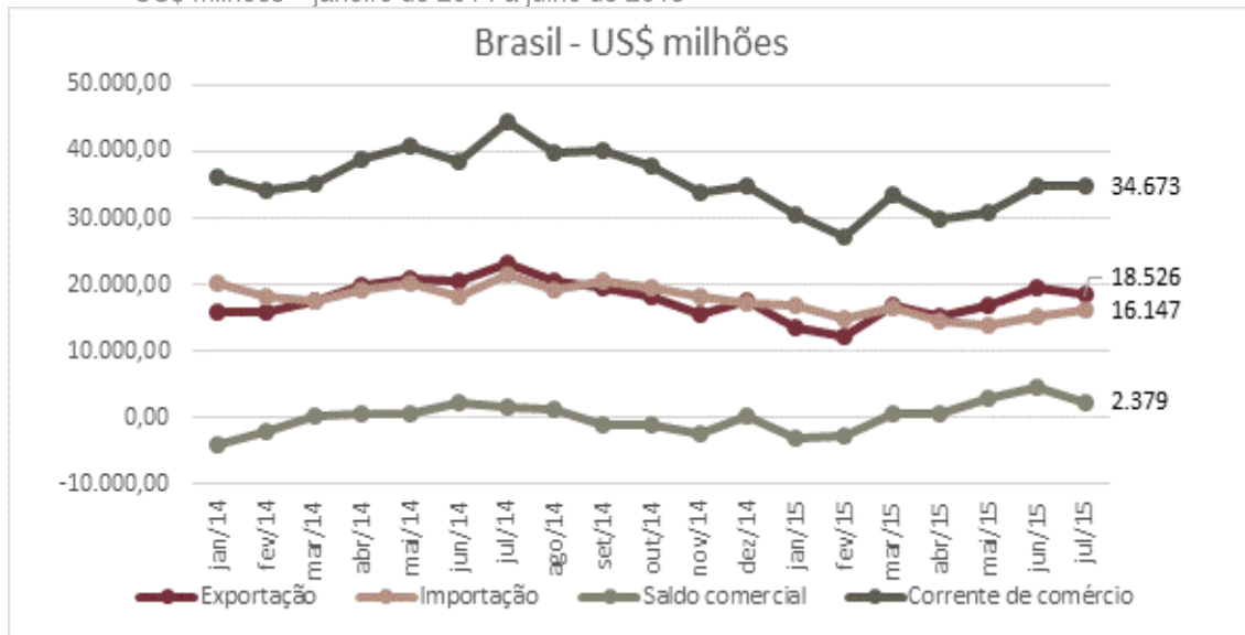
Gráfico 2 - Exportações, Importações, Saldo Comercial e Corrente de Comércio do Brasil US$ milhões – janeiro de 2014 a julho de 2015
